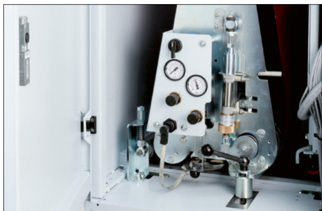
Bedienelemente auf der Bandwechselseite
