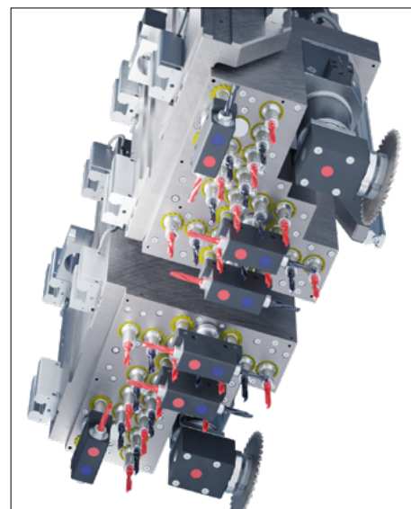
Konfiguration 48-Spindler mit doppeltem Bohrkopf
