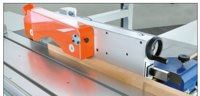
Kreissägen-Vorschubapparat
