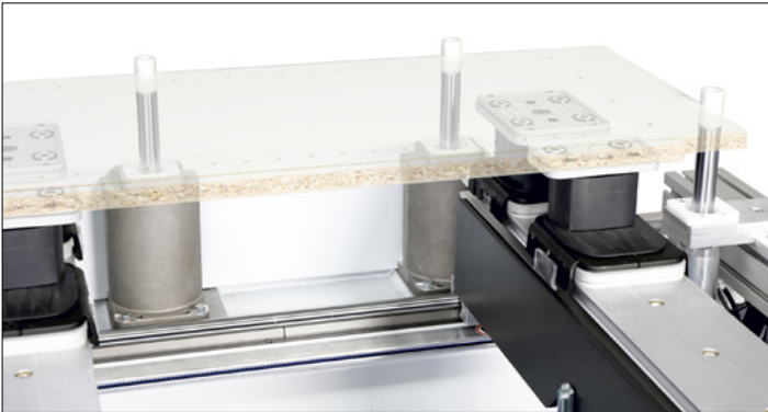
Anschlagsystem hinten, vorne und seitlich
