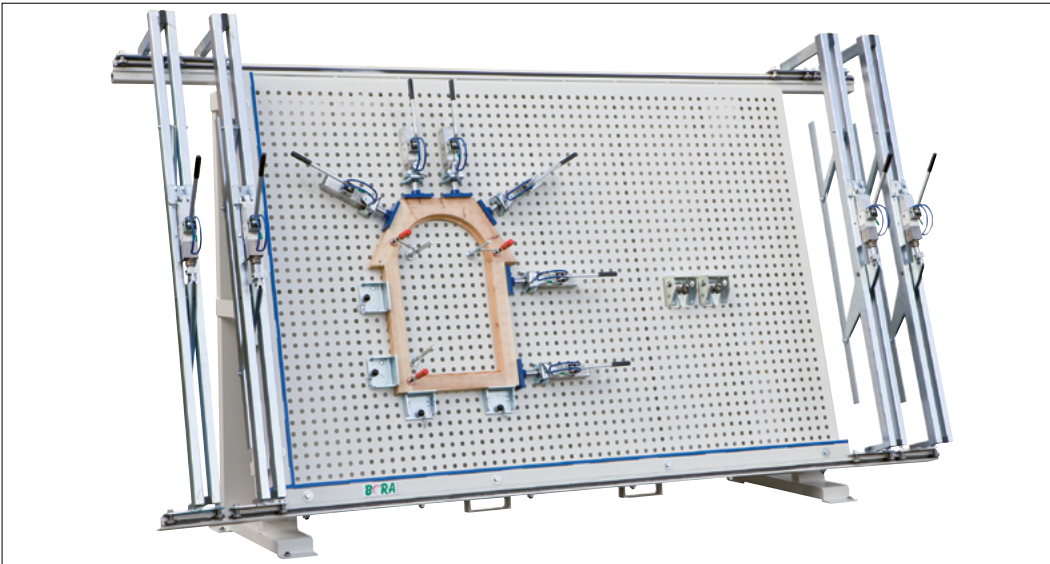
Universal-Lochplattenpresse Beck Bora
