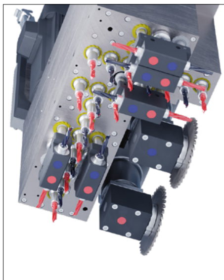
Konfiguration 28-Spindler
