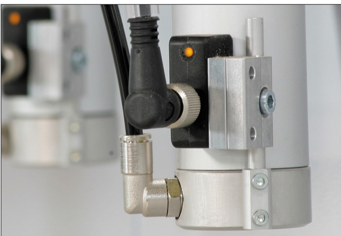
Elektronische Endlagenabfrage
