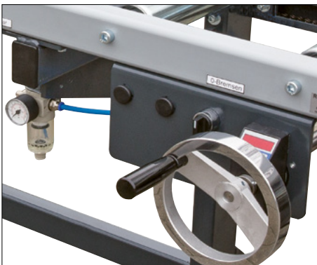
Handradverstellung mit LED-Anzeige in mm, an zentraler Bedienkonsole
