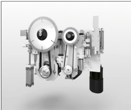
Sägewagen
