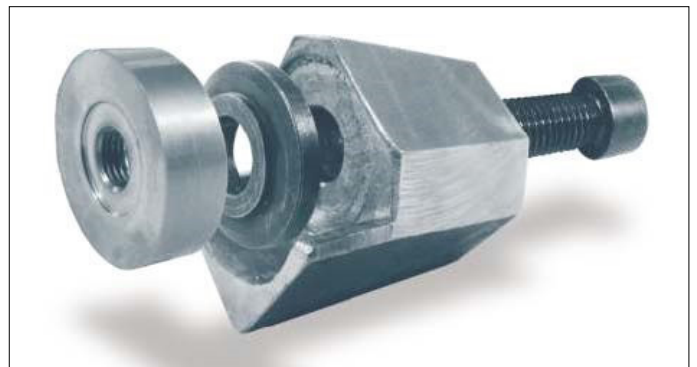
Detail Messersystem Version 7 – Messeraufbau aus Messertträger und Rundmesser
