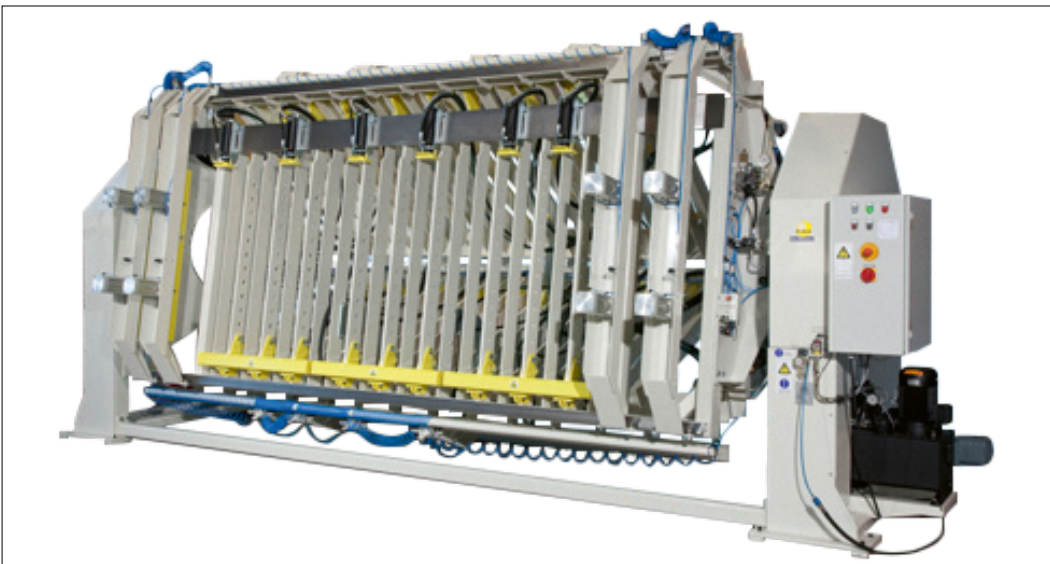
3-Ebenen-Elektrohydraulische Verleimpresse Beck
