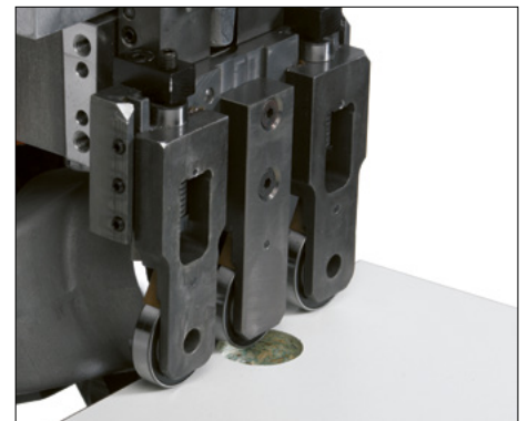
Mehrfachtastrullen
