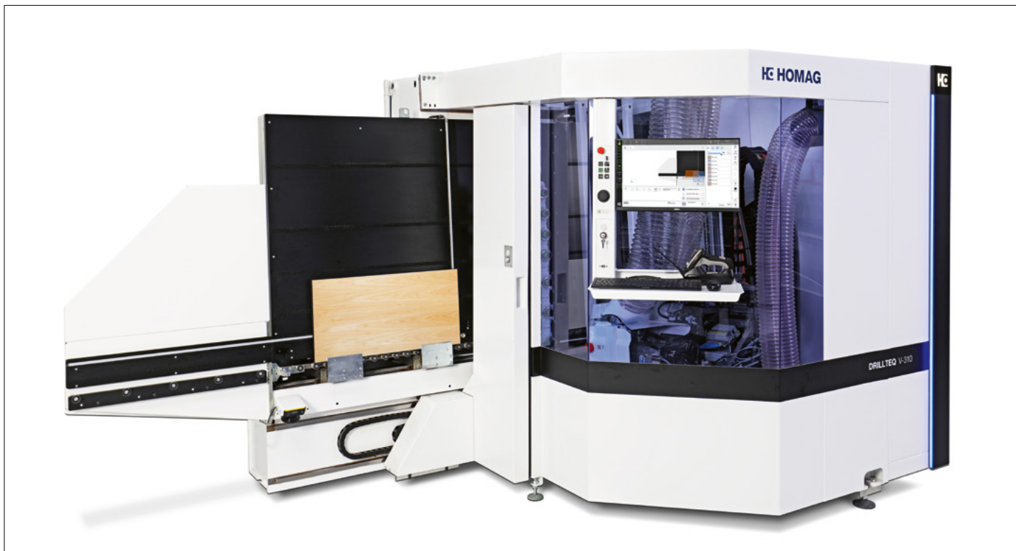
Vertikales CNC-Bearbeitungszentrum HOMAG DRILLTEQ V-310
