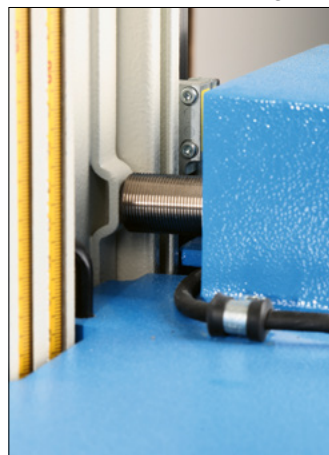
Berührungslose Abstimmung der Rostverstellung
