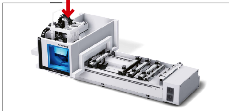
Horizontales CNC-Bearbeitungszentrum HOMAG CENTATEQ P-110 5-Achs
