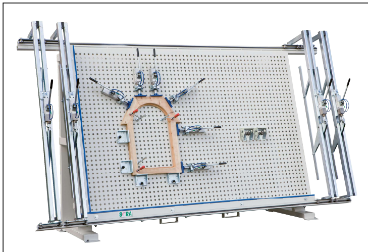
Universal-Lochplattenpresse Beck Bora
