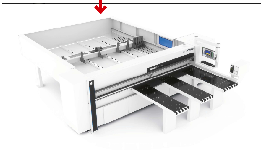
Horizontale Plattenaufteilsäge HOMAG SAWTEQ S-100
