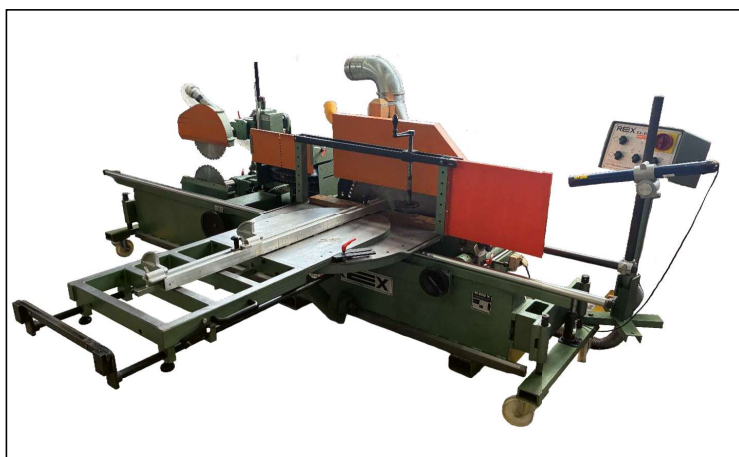
Zapfenschneidmaschine REX ZA800SL
