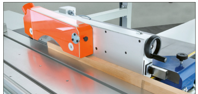
Kreissägen-Vorschubapparat
