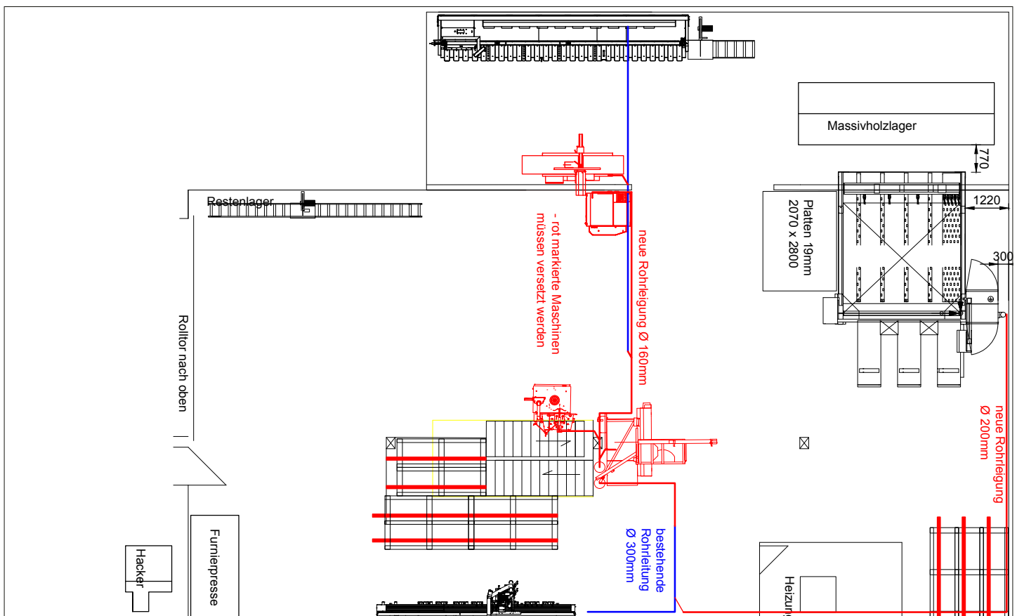
Nach der Planung wurde die Inbetriebnahme einer liegenden Plattenaufteilsäge realisiert
