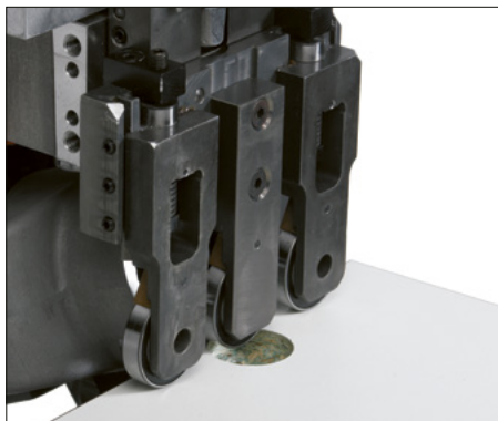
Mehrfachtaastrollen
