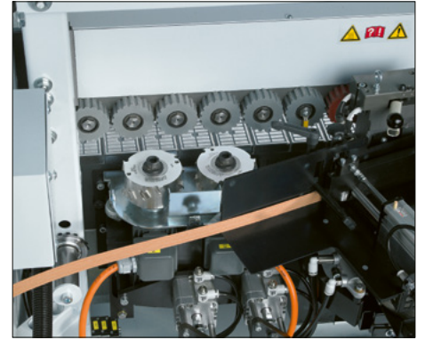
Fügefräsaggregat
