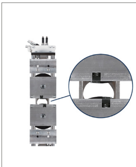
Leimfugenziehklingenaggregat
