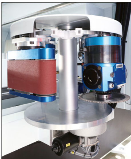
8-fach-Tellerwechsler In X-Richtung, mitfahrend
