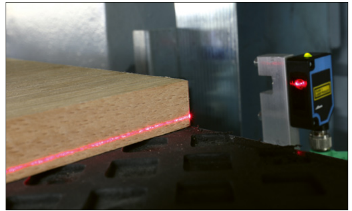
Werkstückdickenmessung
