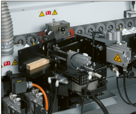
Automatisches Fixlängenmagazin
