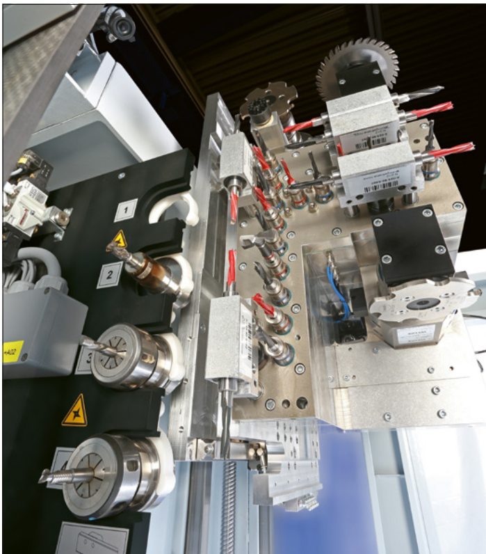
Konfiguration 25-Spindler mit Clamex-Aggregat
