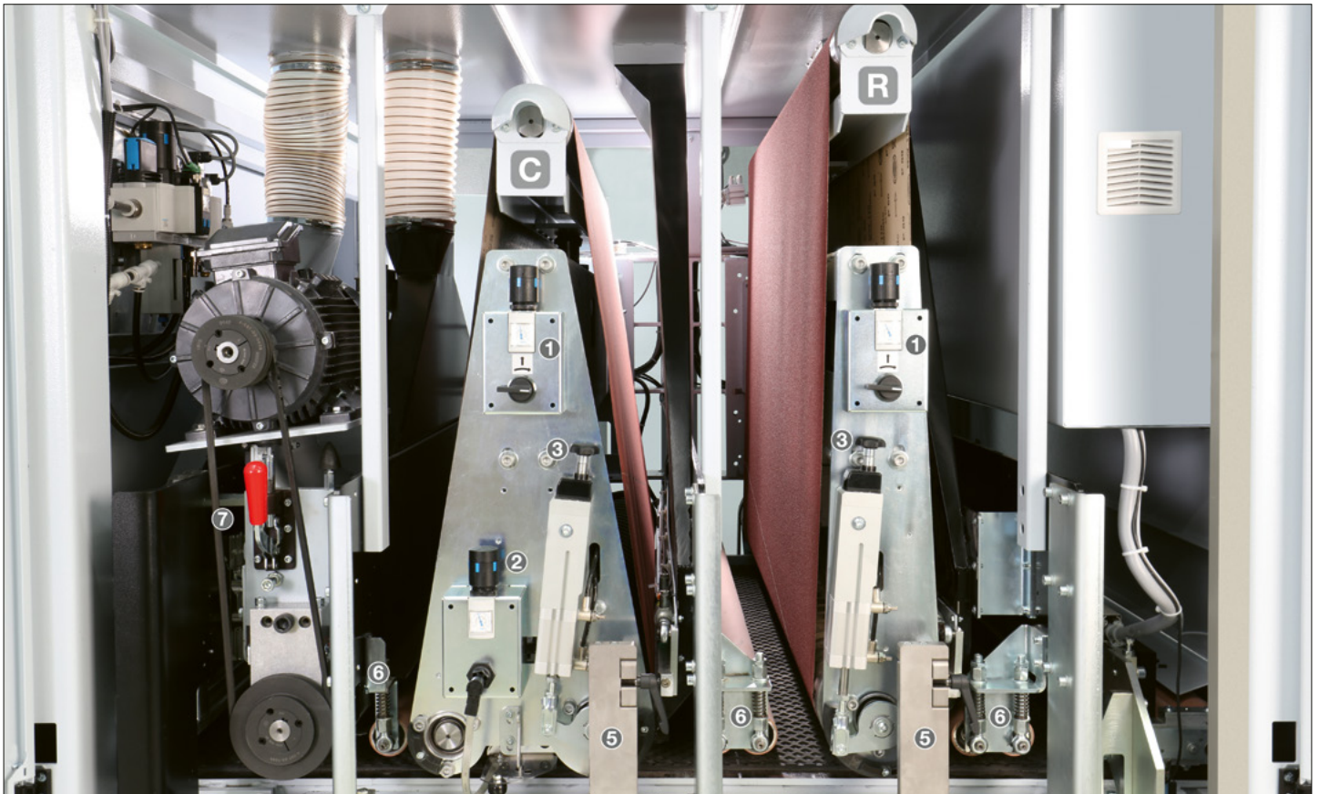
Aggregateanordnung mit Kalibrieraggregat, Kombiaggregat und Bürststation
