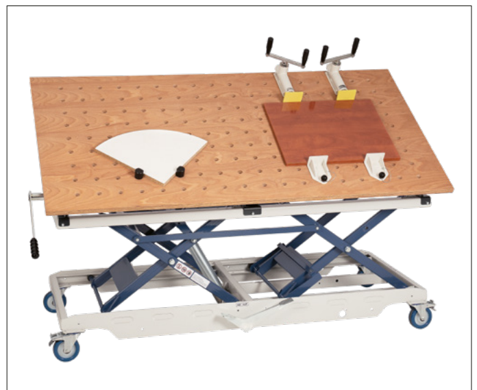
Niveau-Hubtisch Beck HS 300 gross mit Kippeinrichtung und Buchen-Lochraster-Arbeitsplatte, mit Zubehör
