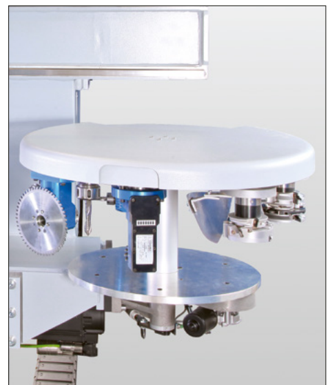
14-fach-Tellerwechsler In X-Richtung, mitfahrend
