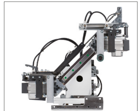
Kappaggregat
