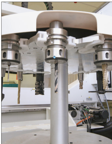
14-fach-Tellerwechsler in X-Richtung, mitfahrend
