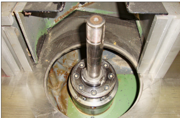
Kehlspindel mit Lagerschaden
