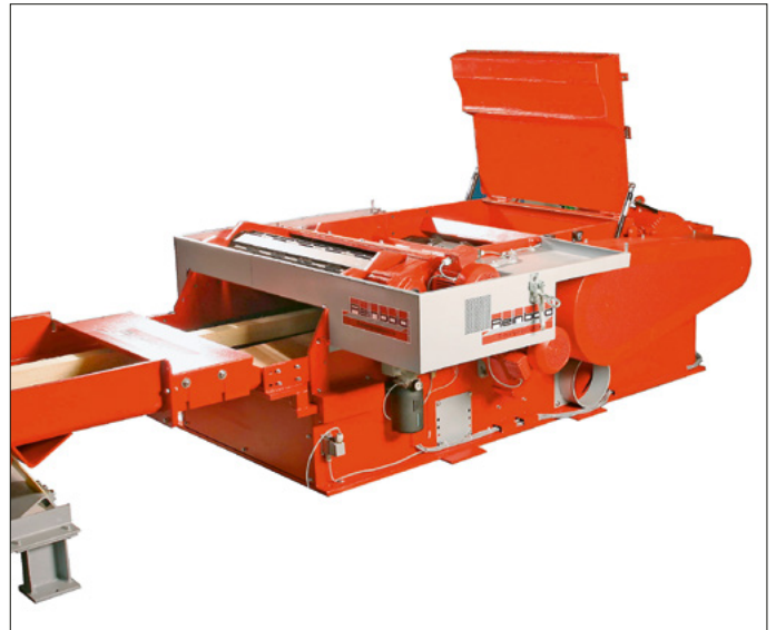
Horizontalzerkleinerer Reinbold RHZ 400 – RHZ 1300 S
