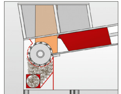
Rotor mit 482 mm Durchmesser für sehr hohen Durchsatz
