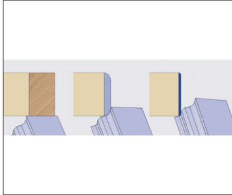
Positionen zum Mehrstufen Fräsaggregat
