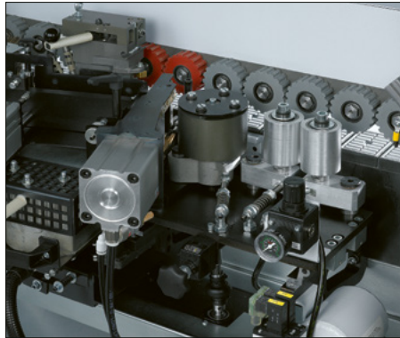
Druckzone
