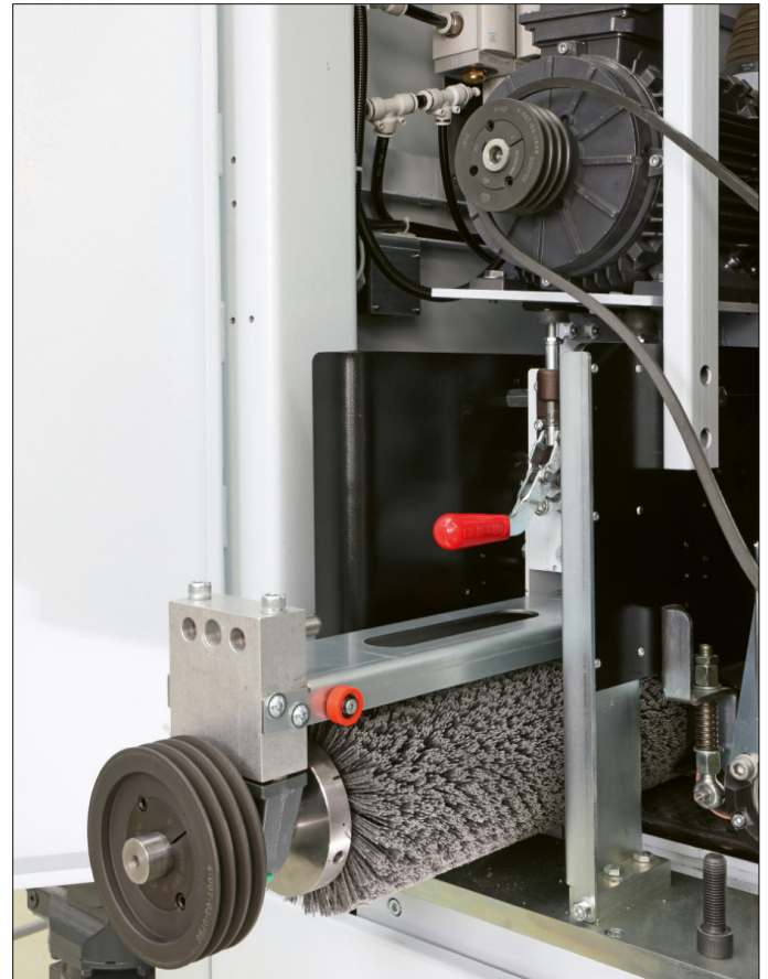
Strukturierbürste Anderlon
