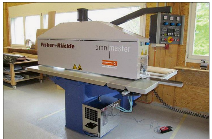
Maschine betriebsbereit aufgebaut
