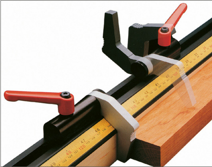
Präzision am laufenden Band – Ein Längenmesssystem, das aus jeder manuellen Bearbeitungsmaschine eine Präzisionsanlage macht, eröffnet im Bereich der Holz-, Metall- und Kunststoffbearbeitung ungeahnte Möglichkeiten – schneller, präziser, wirtschaftlicher.
