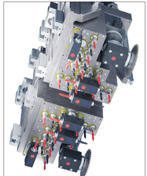
Konfiguration 34-Spindler mit doppeltem Bohrkopf
