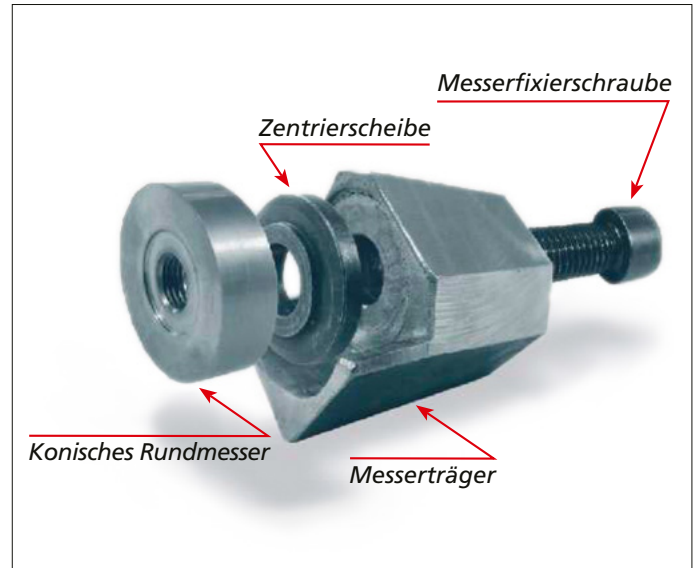
Detail Messersystem Version 7 – Messeraufbau aus Messerträger und Rundmesser
