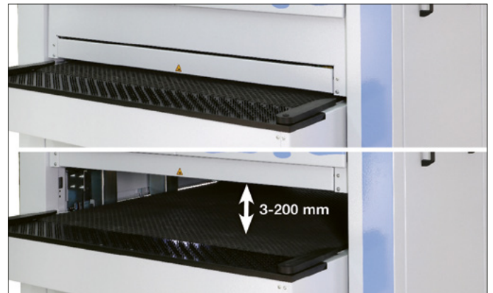
Werkstückdickeneinstellung
