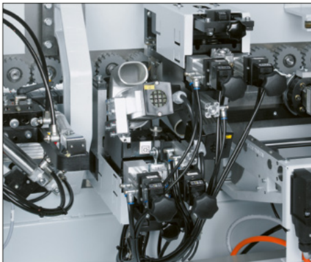
Fräsaggregat mit pneumatischer 3-Punkt-Verstellung
