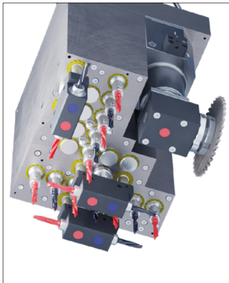
Konfiguration 23-Spindler
