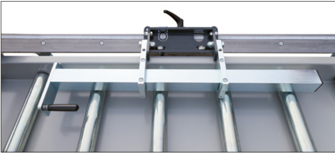
Manuell verstellbarer Anschlagwagen mit analogem Messsystem und Ableselupe
