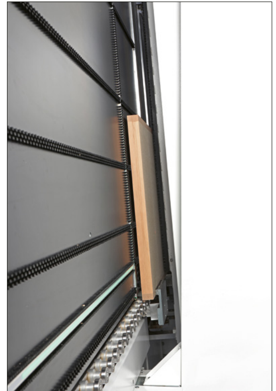
Werkstückhandling mit 5 Grad Neigung
