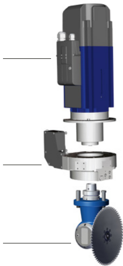
CNC-Bearbeitungszentrum HOMAG CENTATEQ P-110, 4-Achs-Variante
