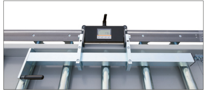
Manuell verstellbarer Anschlagwagen mit digitaler Massanzeige
