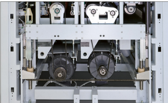
Massive Rahmenkonstruktion
