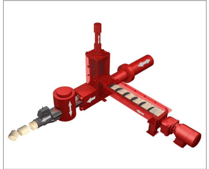
Funktionsschema
