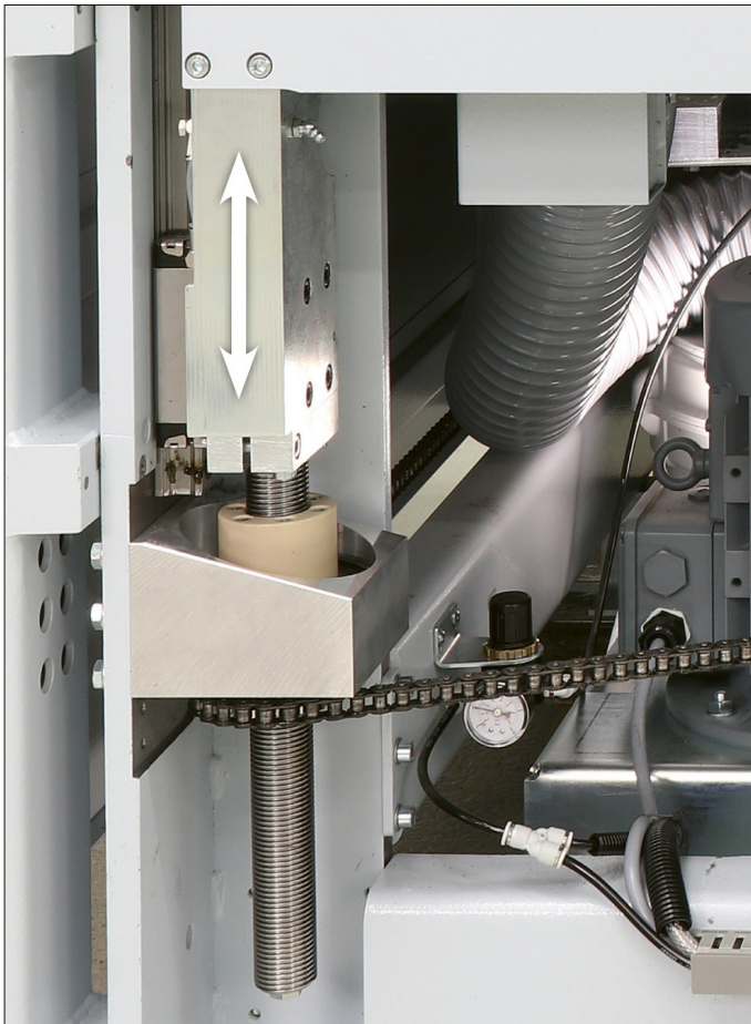
Massive Konstruktion der Höhenverstellung
