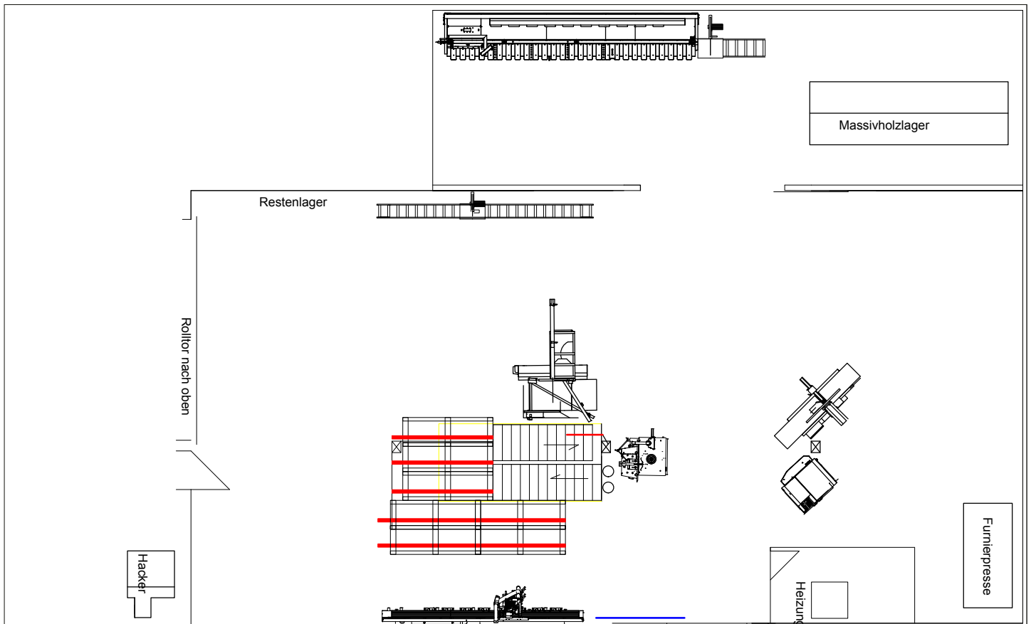
Ist-Zustand eines Betriebs mit vertikalem Plattenzuschnitt
