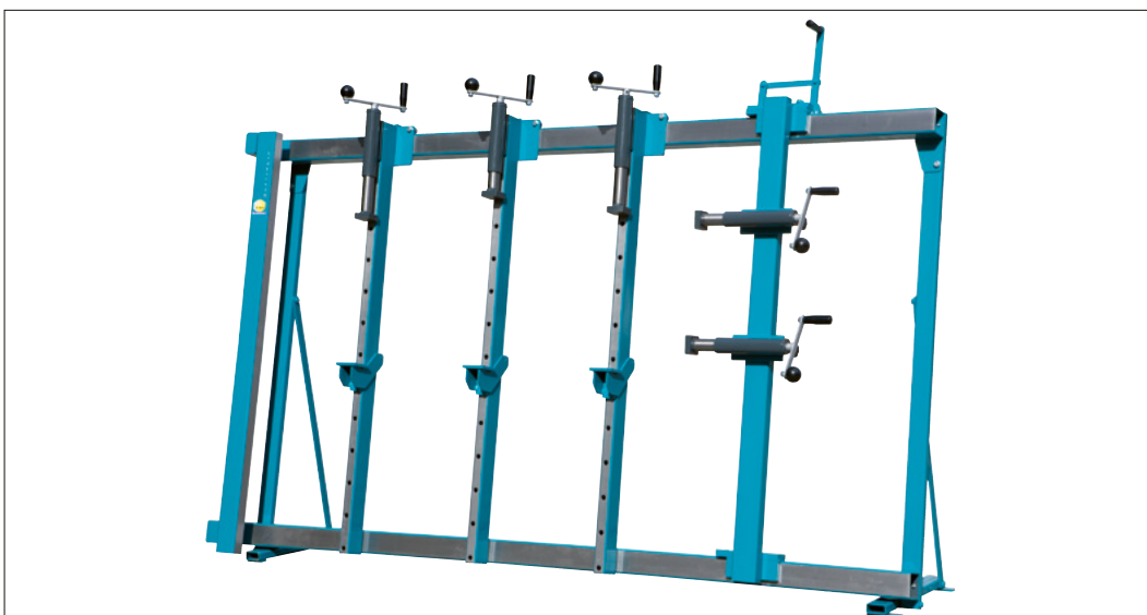
Verleimpresse Beck Quattrra LC
